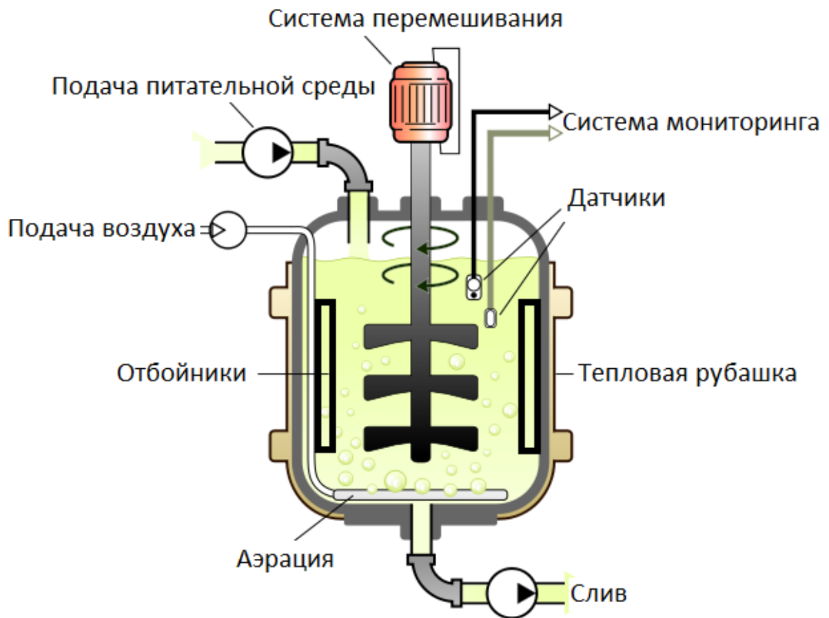
Рисунок 4.3 – Схема ферментера
