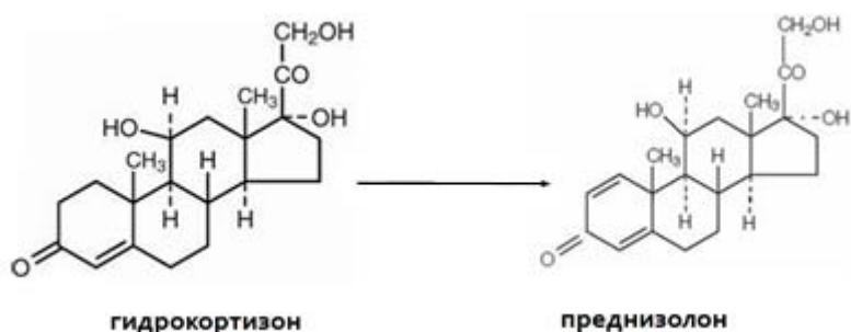
Рисунок 21.3 – Биотрансформация гидрокортизона в преднизолон
