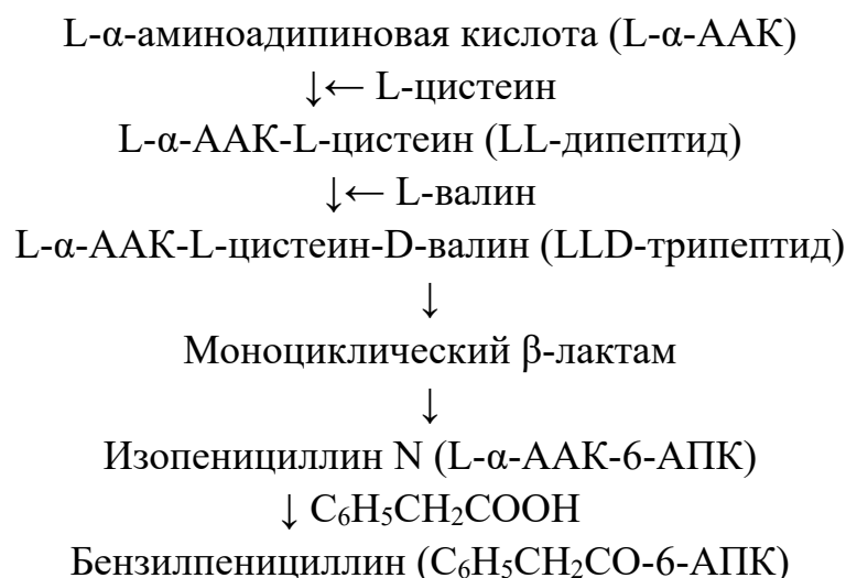
Рисунок 22.1 - Схема биосинтеза молекулы пенициллина
