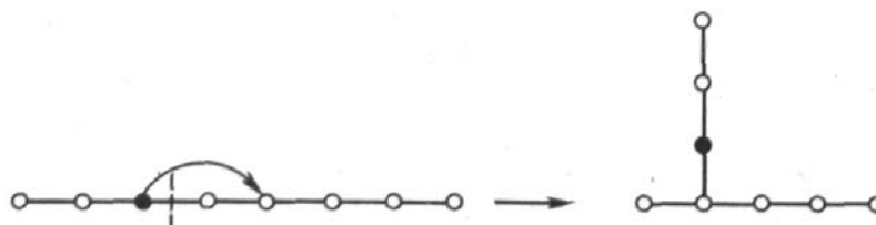
Рисунок 18.2 – Схема образования гликозидной связи
