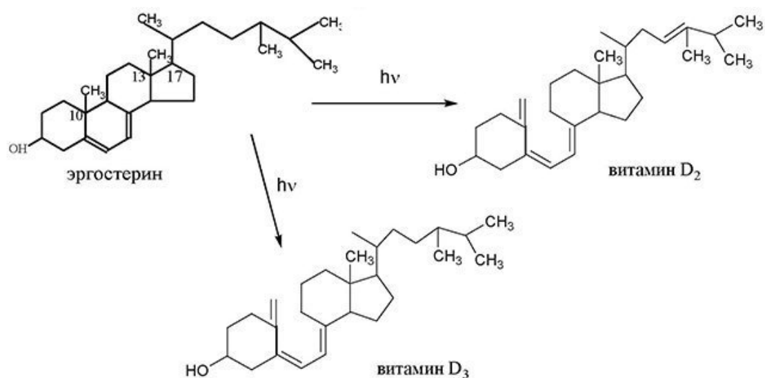
Рисунок 16.3 – Превращение эргостерина под действием УФ-излучения
