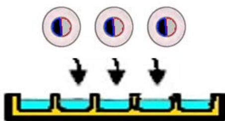
Рисунок 12.3 – Первое клонирование гибридных клеток на полной культуральной среде
